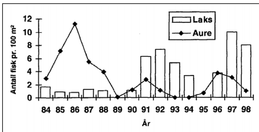
Figur 41. Tetthet av laks- og ørretunger eldre enn årsyngel i Aureelva i perioden 1984-1998. Gyrodactylus salaris ble påvist 1984 og vassdraget ble rotenonbehandlet i 1988. Fra Johnsen et al. (1999).
