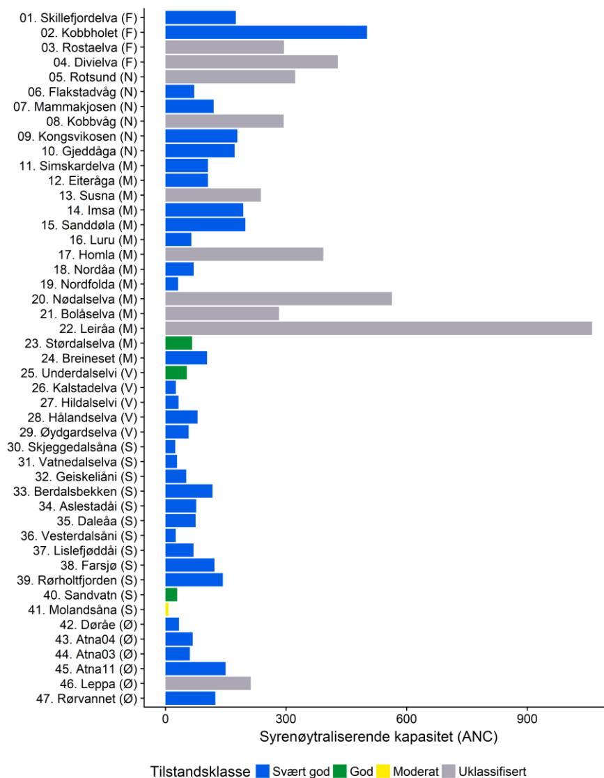
Figur 18. Tilstandsklassifisering av forsurningsparameteren syrenøytraliserende kapasitet, ANC ( \mu\text{Eq/L} ), for elvene som var med i overvåkingen i 2017. Søylen viser gjennomsnittsverdier ANC. Fargen indikerer tilstandsklassen. Merk: typespesifikke klassegrenser.
