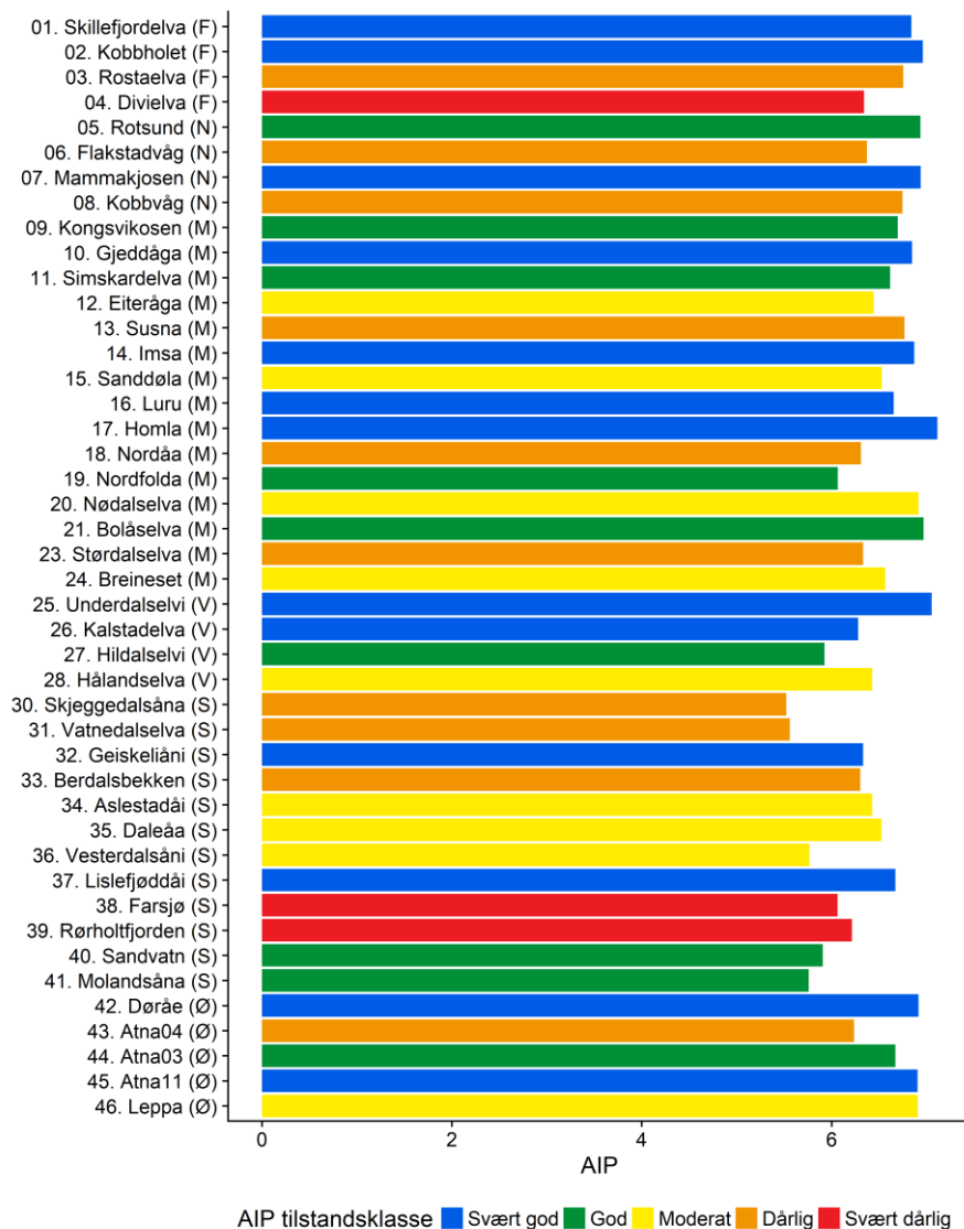
Figur 6. Indeksverdier for forsøringsindeksen for påvekstalger (AIP) for de 46 undersøkte vannforekomstene i 2017, inkludert moderat kalkrike vannforekomster. I Rørvannet og Leiråa var det for få indikatorarter til sikker klassifisering og disse er derfor ikke inkludert i figuren. Fargene viser tilstandsklasse. Merk: typespesifikke klassegrenser
