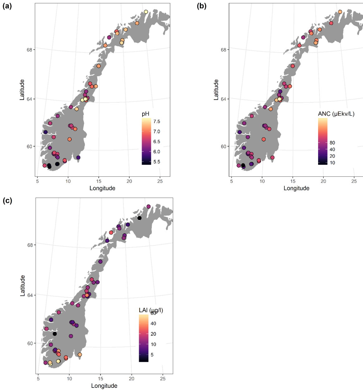
Figur 16. Midlere verdier av pH (a), ANC(b) og maksimumsverdier av LAl (c) i de ulike vannforekomstene.
