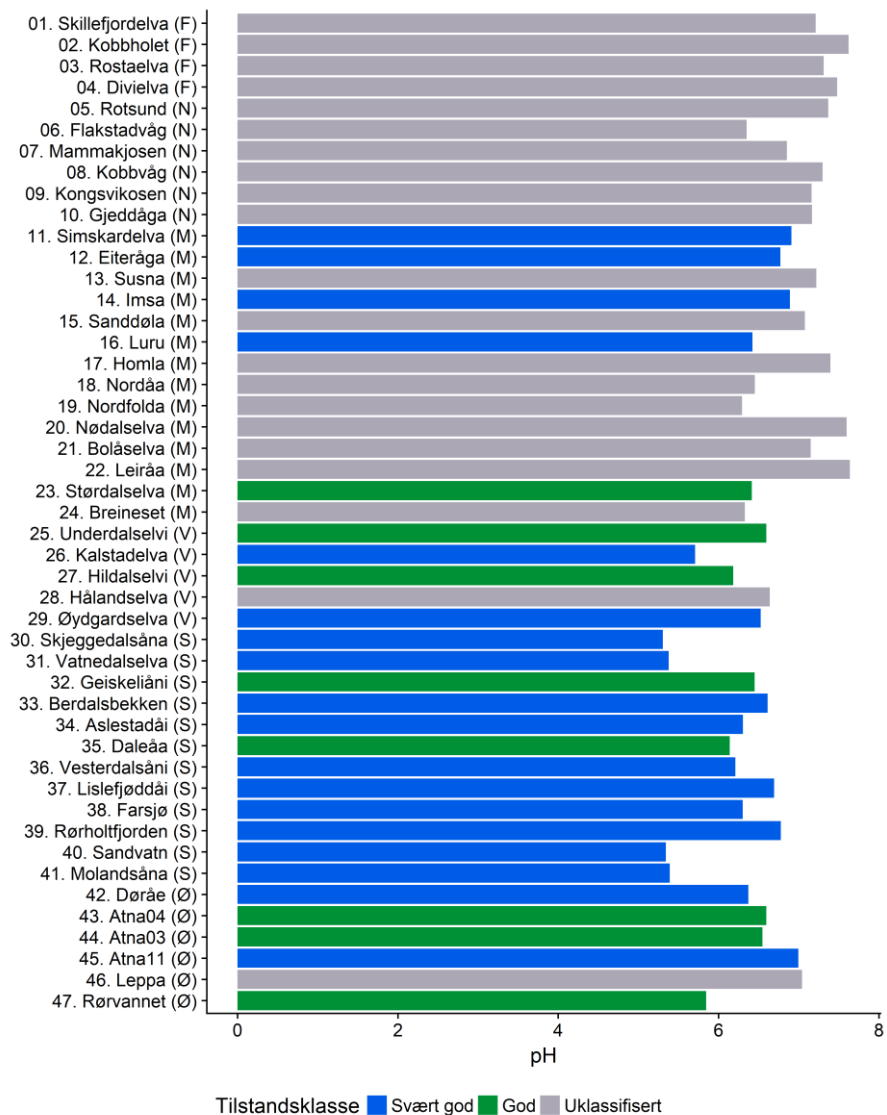
Figur 17. Tilstandsklassifisering av forsurningsparameteren pH for elvene som var med i overvåkingen i 2017. Søylen viser gjennomsnittsverdier for pH. Fargen indikerer tilstandsklassen. Grå søyler markerer moderat kalkrike og/eller anadrome vannforekomster. Merk: typespesifikke klassegrenser.
