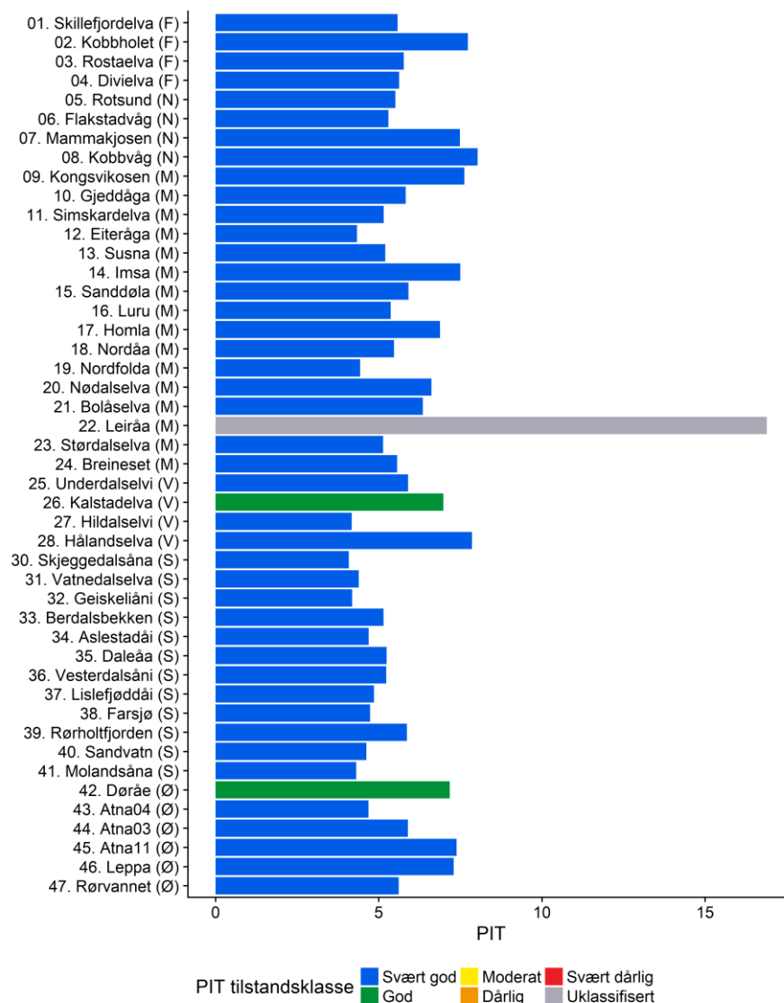
Figur 5. Indeksverdier for eutrofieringsindeksen for påvekstlger (PIT) for de 46 undersøkte vannforekomstene i 2017. Da det ikke er utviklet klassegrenser for leirvassdrag kan vi ikke tilstandsklassifisere Leiråa, og denne har derfor grå søyle. Fargene viser tilstandsklasse. Merk: typespesifikke klassegrenser
