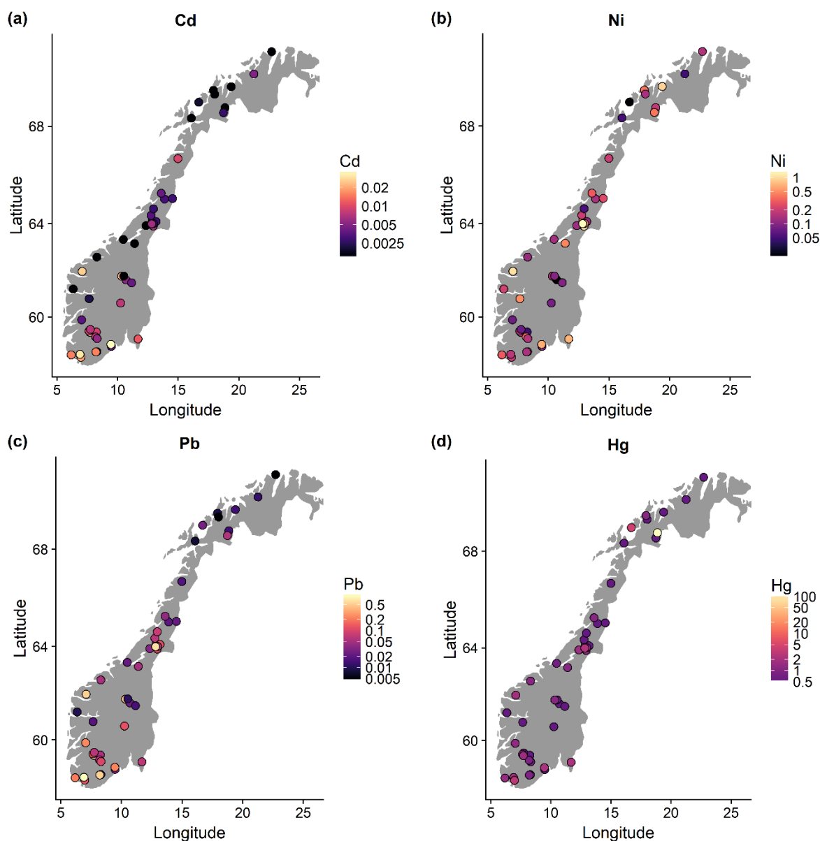
Figur 27. Gjennomsnittskonsentrasjoner (µg/l) av prioriterte stoffer (Cd = kadmium, Ni = nikkel, Pb = bly og Hg = kvikksølv) i vann i de 47 vannforekomstene undersøkt i 2017.
