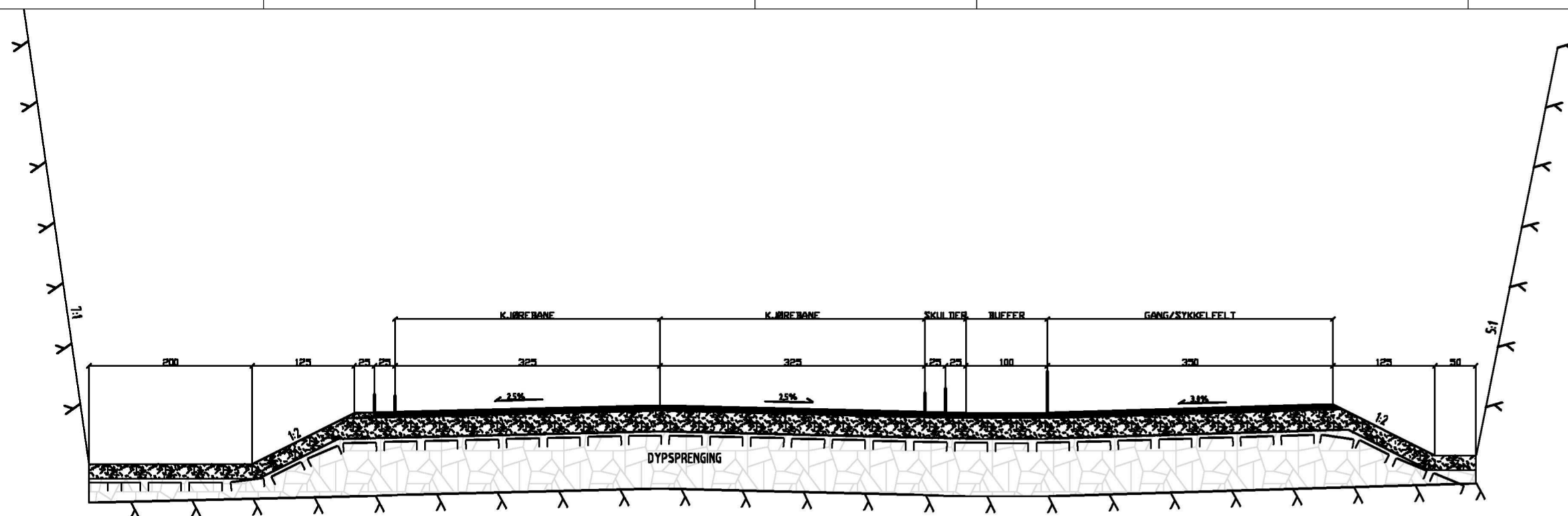
NORMALPROFIL 0-510M
